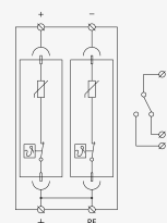
Schéma zapojení
