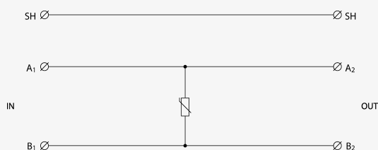
Schéma zapojení
