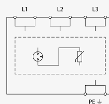
Schéma zapojení
