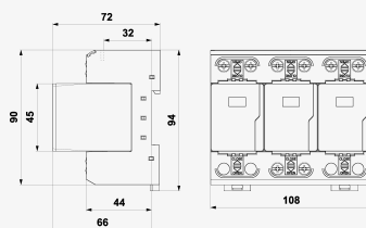
Rozměry
