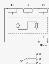
Schéma zapojení
