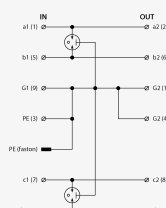
Schéma zapojení
