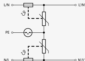
Schéma zapojení
