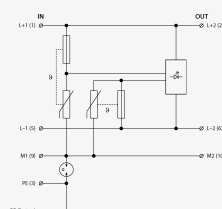
Schéma zapojení
