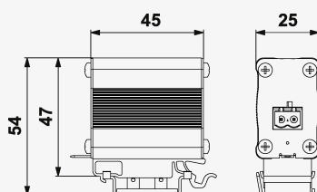
Rozměry
