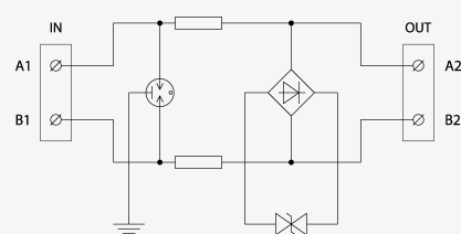
Schéma zapojení
