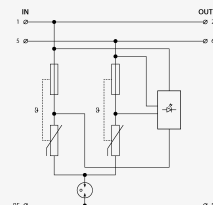
Schéma zapojení
