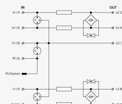
Schéma zapojení
