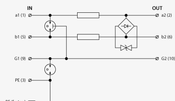
Schéma zapojení
