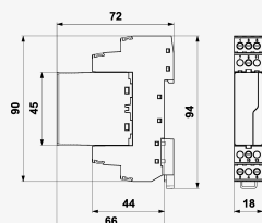
Rozměry
