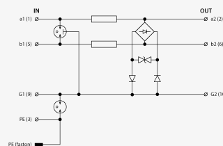
Schéma zapojení
