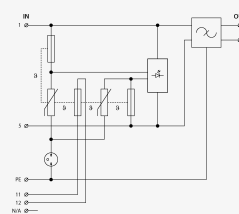
Schéma zapojení
