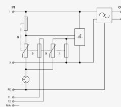
Schéma zapojení
