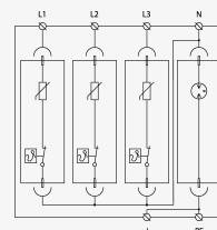
Schéma zapojení
