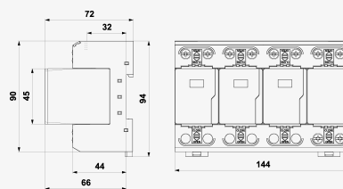
Produktabmessungen
