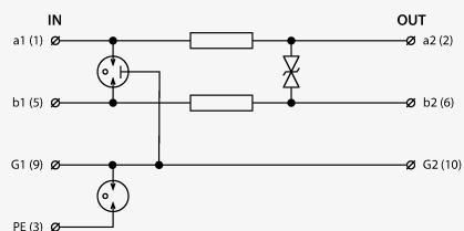
Prinzipschaltbild
