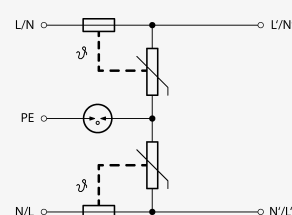
Prinzipschaltbild
