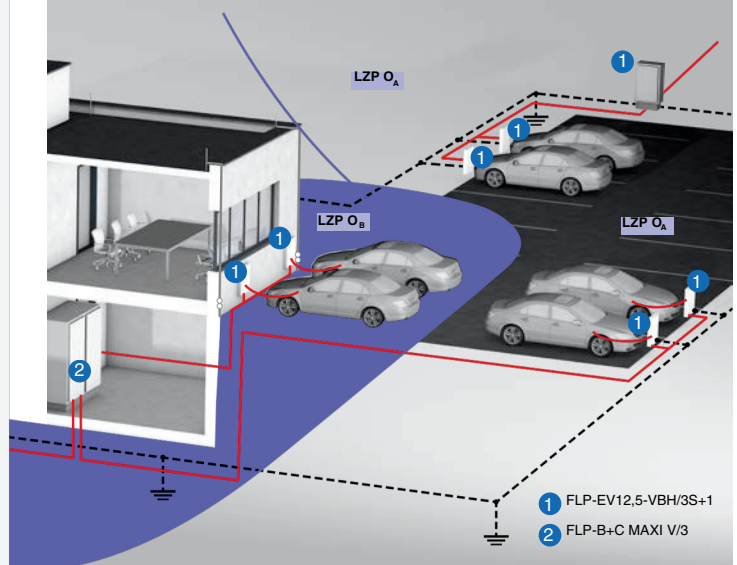
obr. 3 Výběr SPD podle zón ochrany před bleskem
