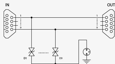
Schéma zapojenia
