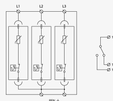
Schéma zapojenia
