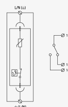
Schéma zapojenia
