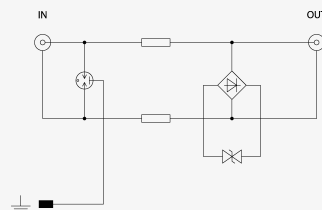
Schéma zapojenia
