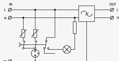
Schéma zapojenia
