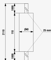
Rozmery produktu
