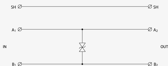
Schéma zapojenia
