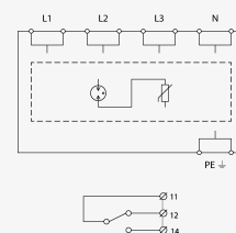
Schéma zapojenia
