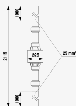
Rozmery produktu
