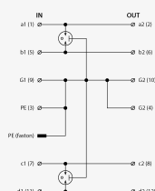
Schéma zapojenia
