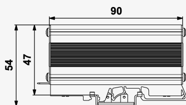
Rozmery produktu
