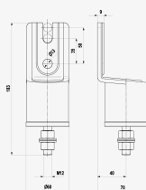
Rozmery produktu
