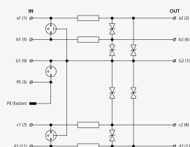
Schéma zapojenia
