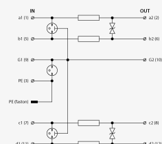
Schéma zapojenia
