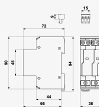
Rozmery produktu
