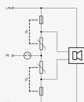
Schéma zapojenia
