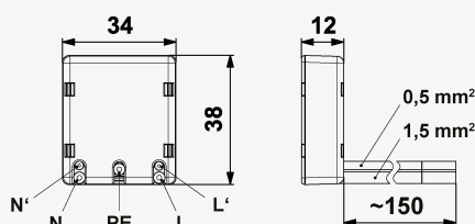
Rozmery produktu
