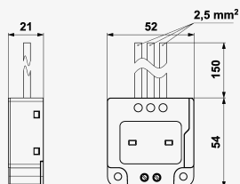
Rozmery produktu
