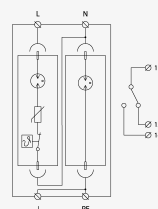
Schéma zapojenia
