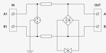
Schéma zapojenia
