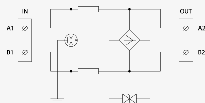
Schéma zapojenia
