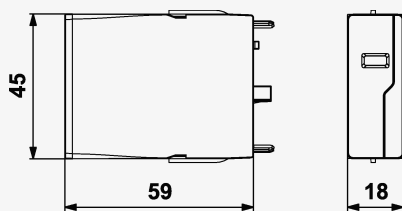
Rozmery produktu
