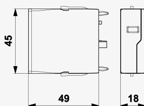
Rozměry produktu
